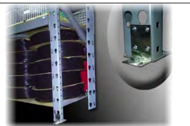
חיבור של רגל קדמית של ארון מחסן למניעת החלקה. (ת)
